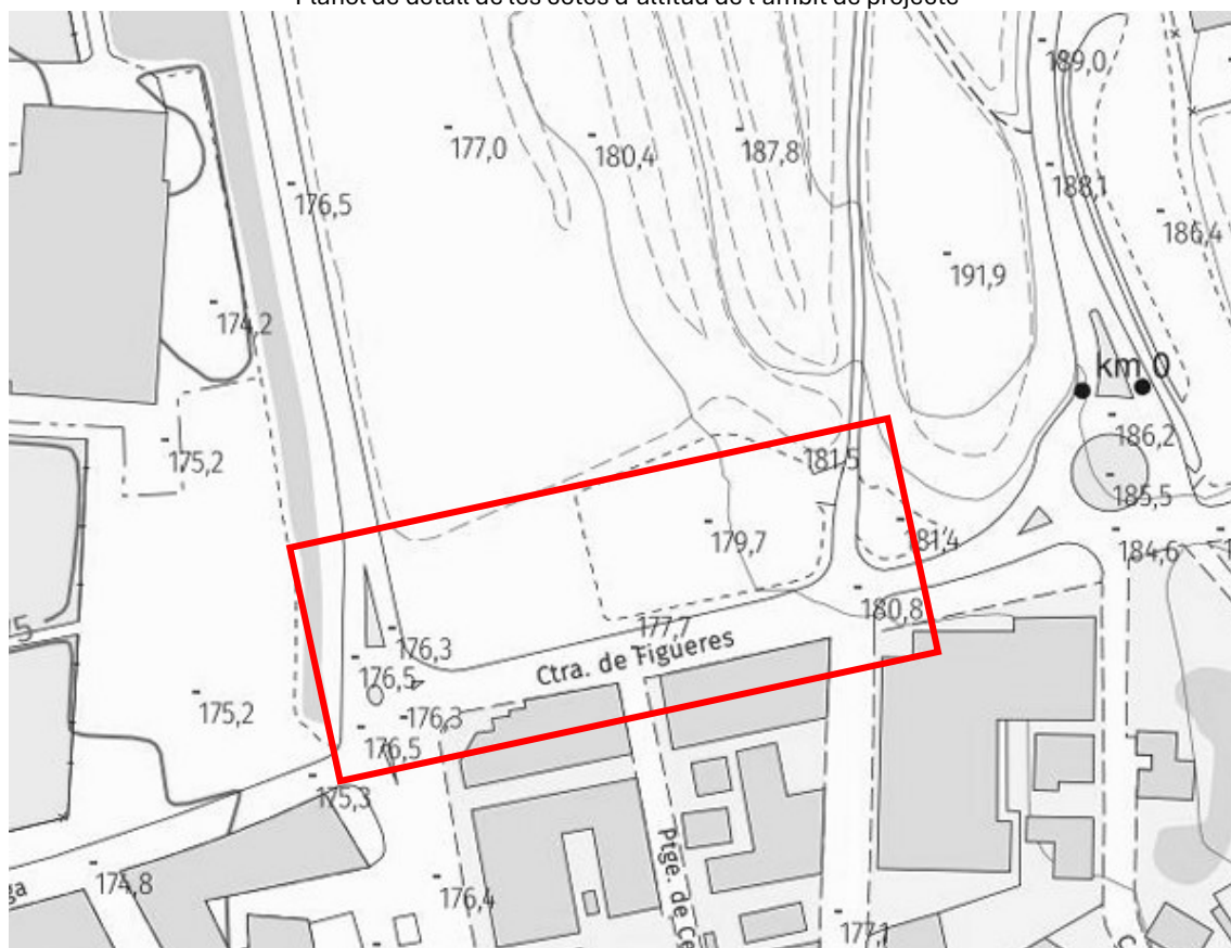
Plànol de detall de les cotes d'altitud de l'àmbit de projecte
